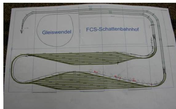
Beispiel von zwei Gleisharfen (FE 2010)
